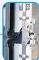
Double-articulation et tringlerie inox
